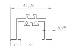
Perfil Opticas
