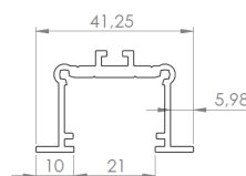
Perfil Difusor
